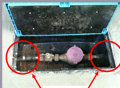
鉛製給水管
